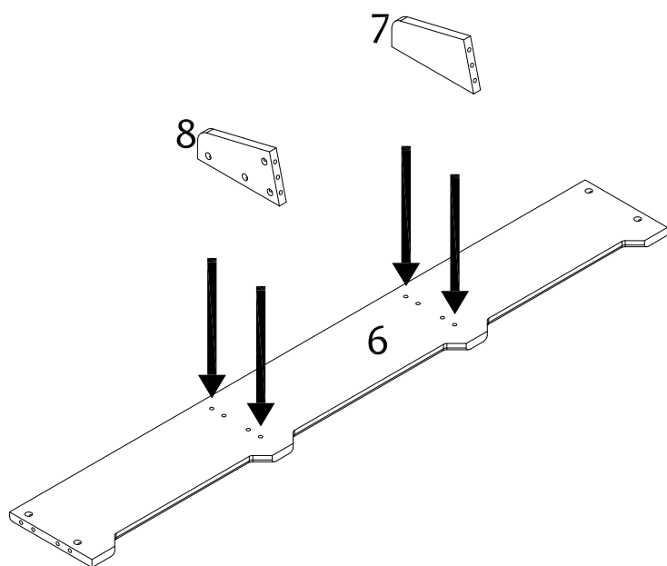
STEP 18
